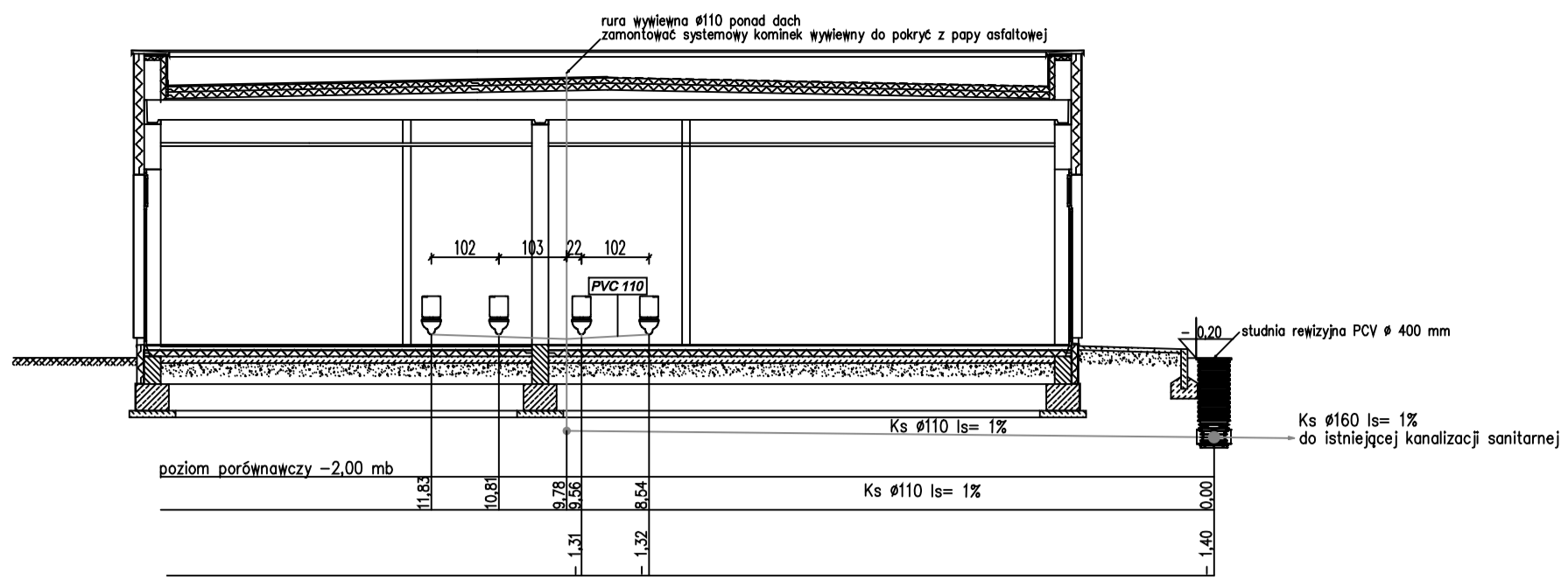
ROZWIŃCIE KANALIZACJI SANITARNEJ skala 1:100
